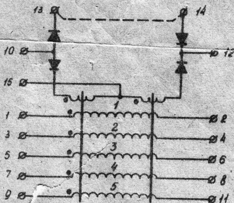
Элемент МР-40Т.
