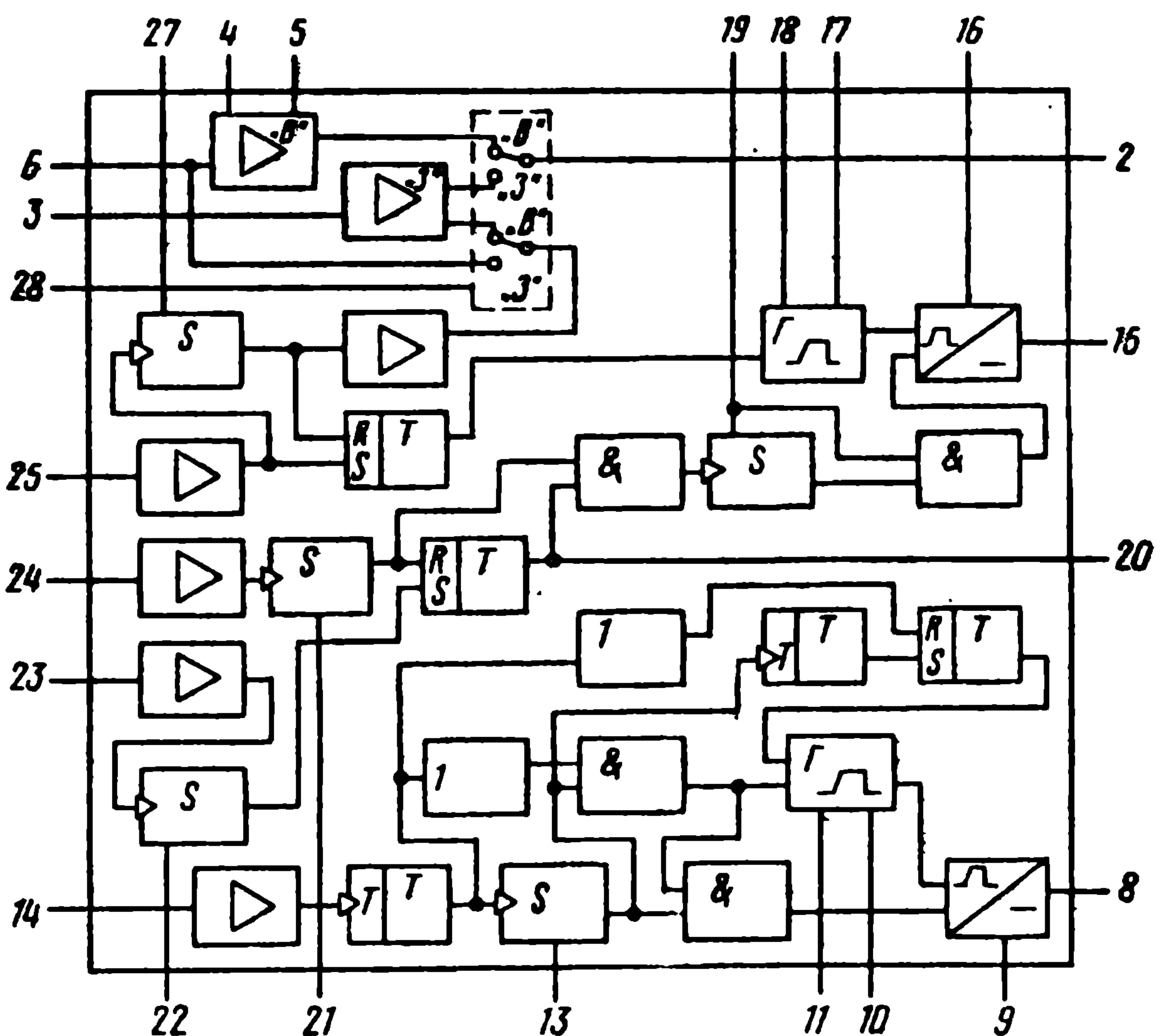
Функциональная схема КР1005ХА2
