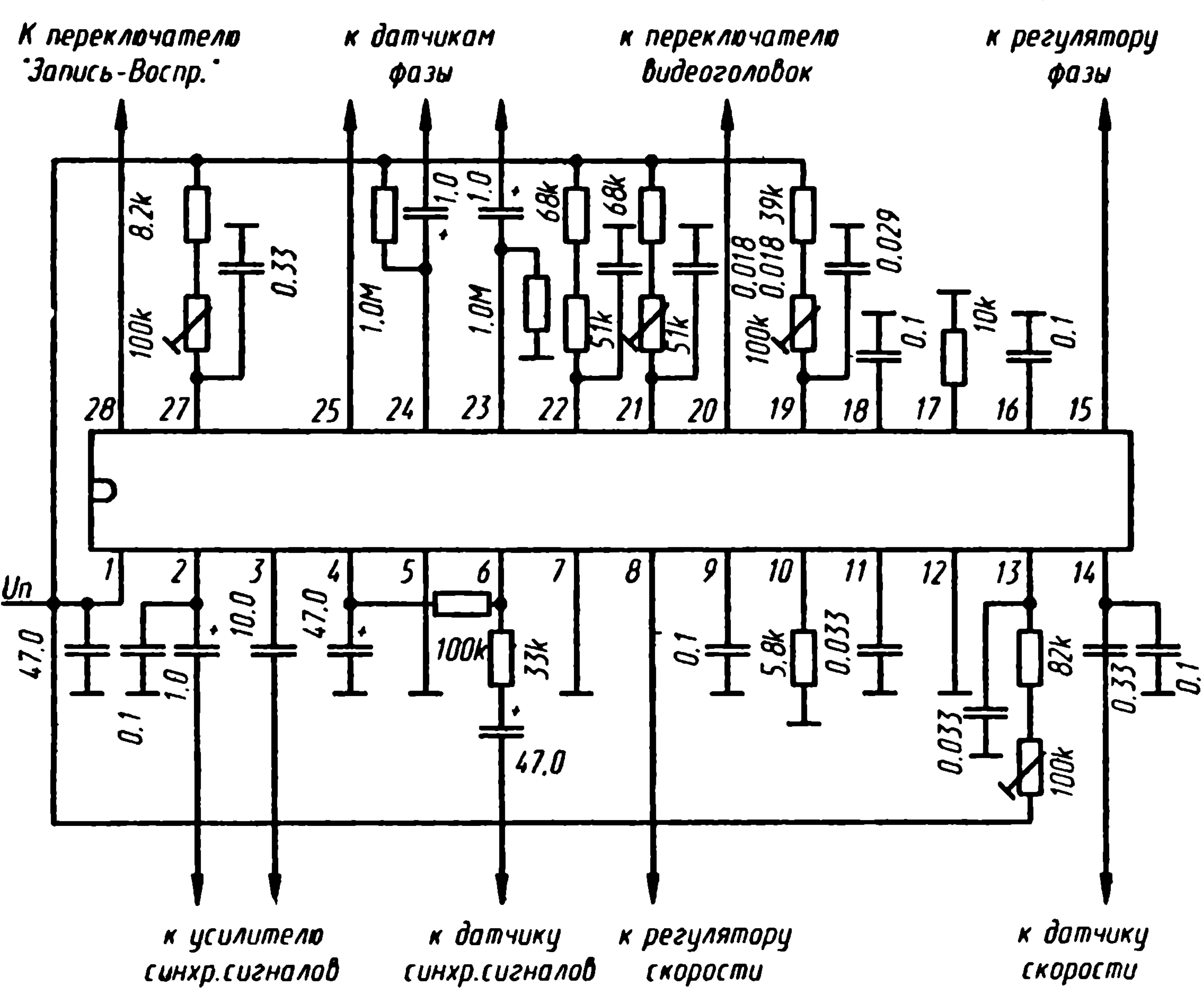
Типовая схема включения КР1005ХА2
