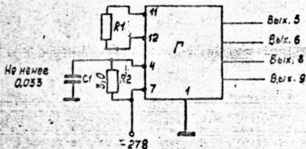
Рис. 1 Схема включения микросхемы К1ГФ651
