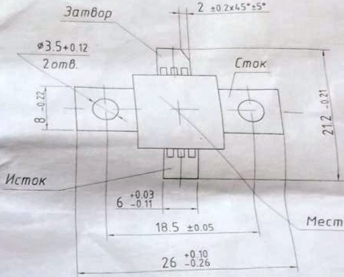
Схема соединения электродов с выводами
