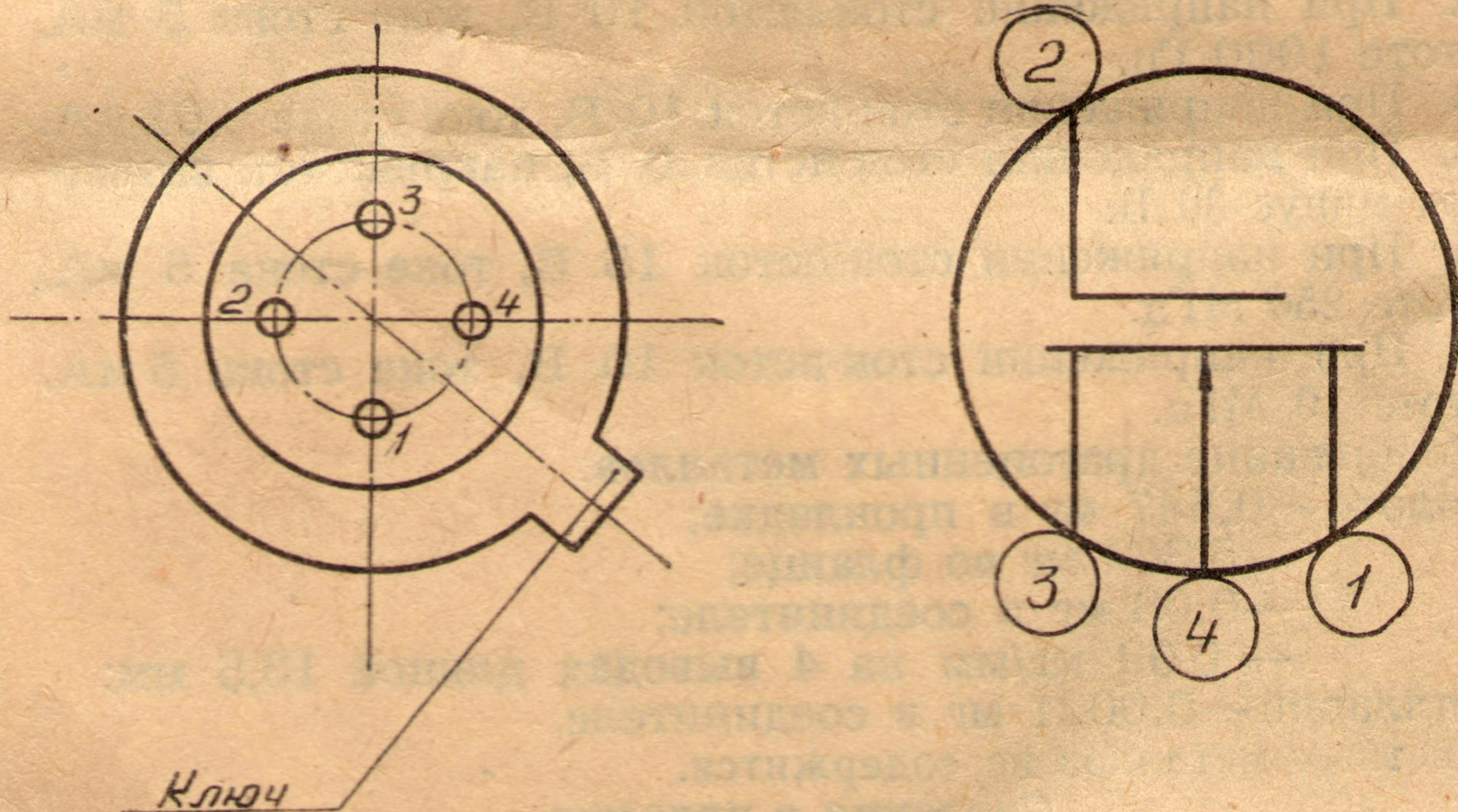
Схема расположения выводов
