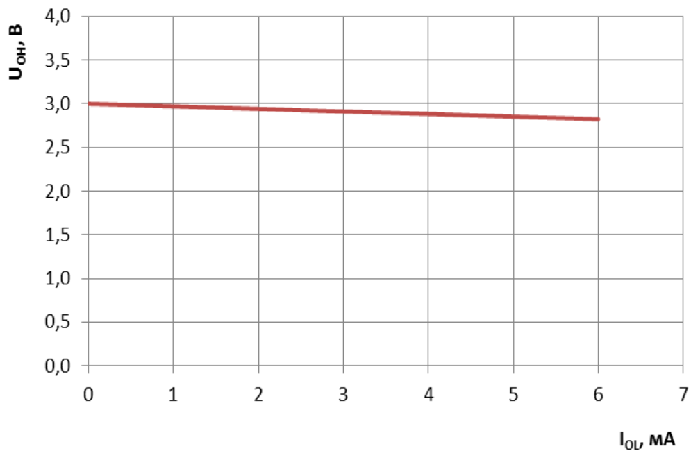
Рисунок 141 – Зависимость выходного напряжения высокого уровня от выходного тока высокого уровня при напряжении питания 3,0 В
