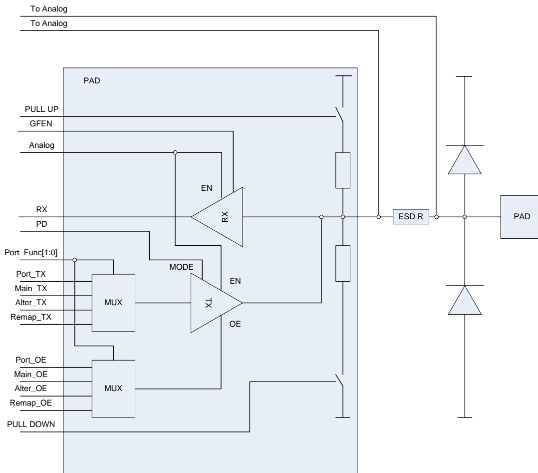
Рисунок 26 – Порты ввода/вывода
