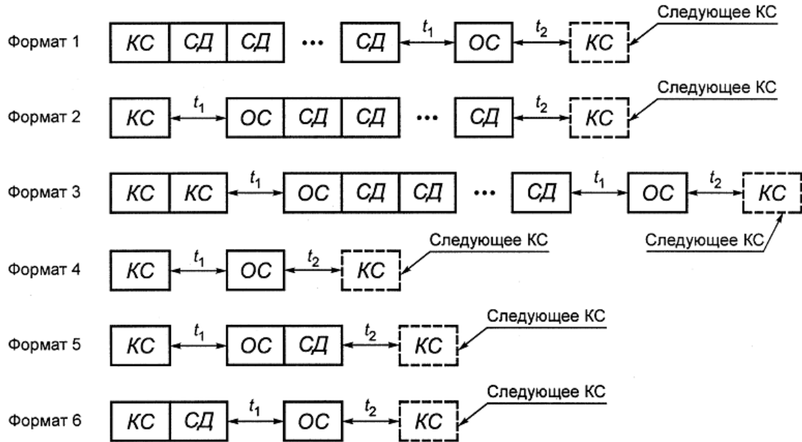
Рисунок 57 – Форматы сообщений
