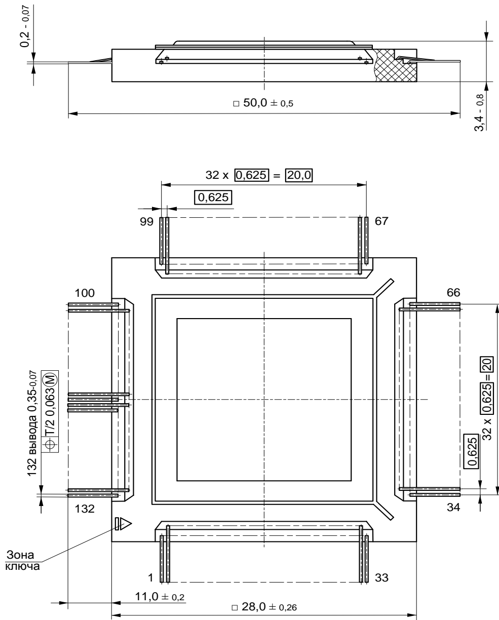
Рисунок 143 – Корпус 4229.132-3
